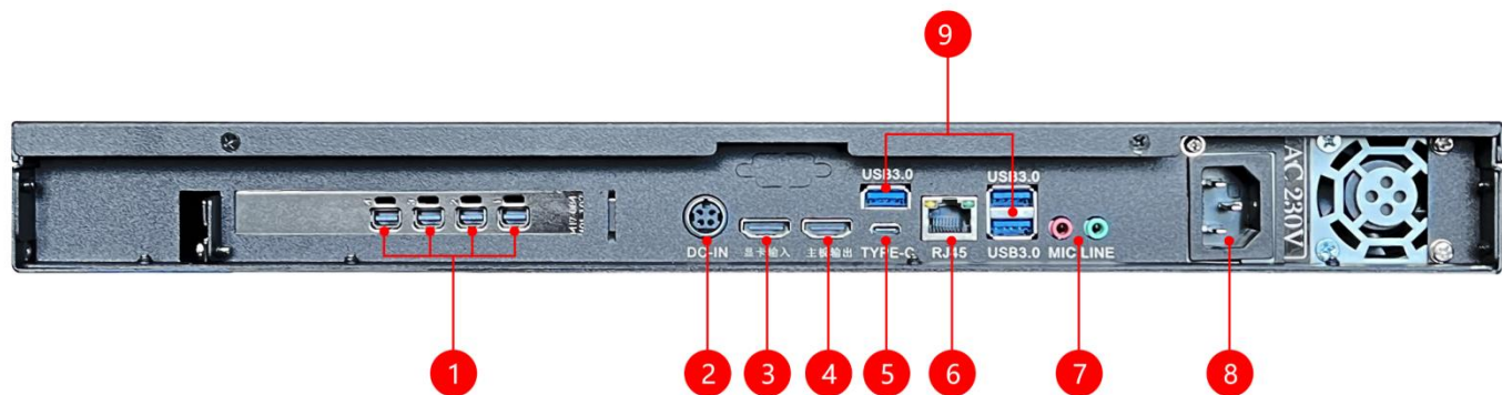
后面板
