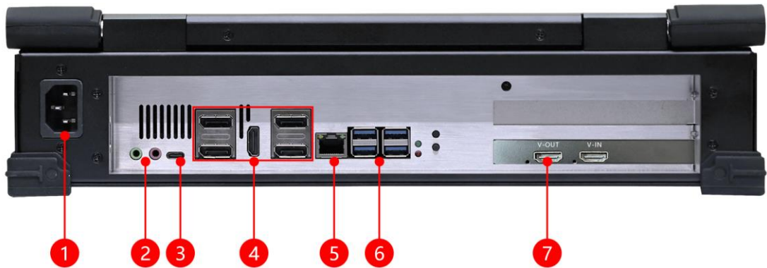
后面板
