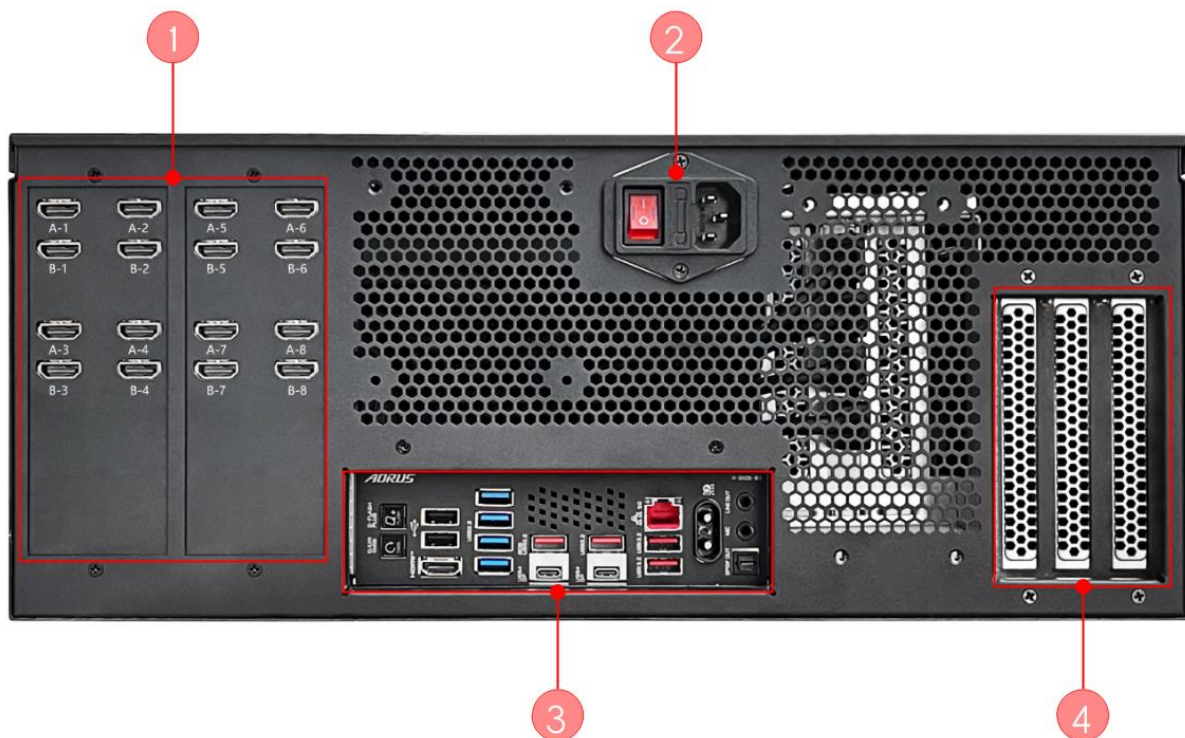
后面板
