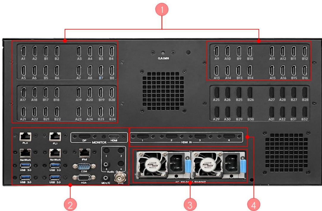
后面板
