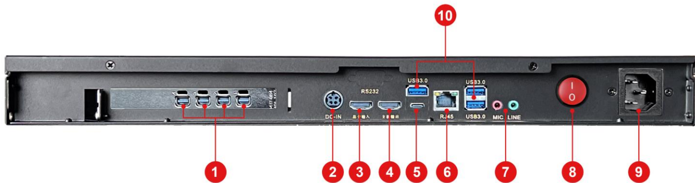
后面板
